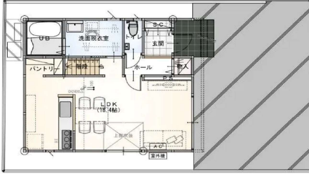
1階 平面図 S:1/100
